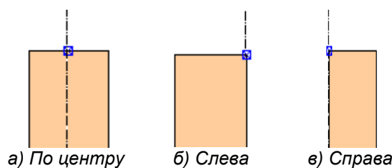
Рис. 3.2 Расположение бруса.
