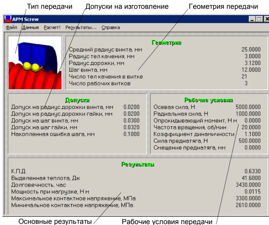
Рис. 2.1 Общий вид системы APM Screw.
